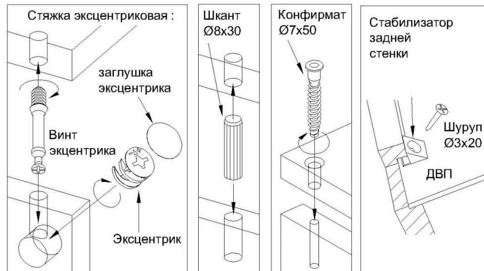
Схема основных крепежных узлов
