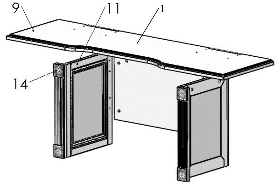
Рисунок 3 – Сборка царги с вертикальными стенками тумб и столешницей
