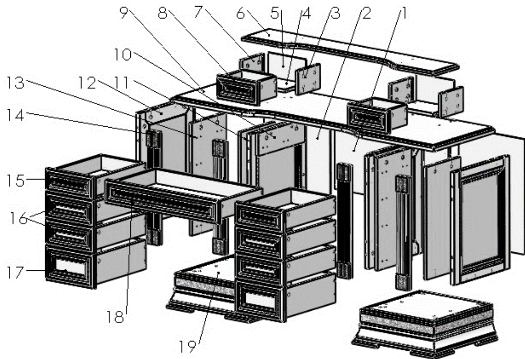
Перечень деталей
