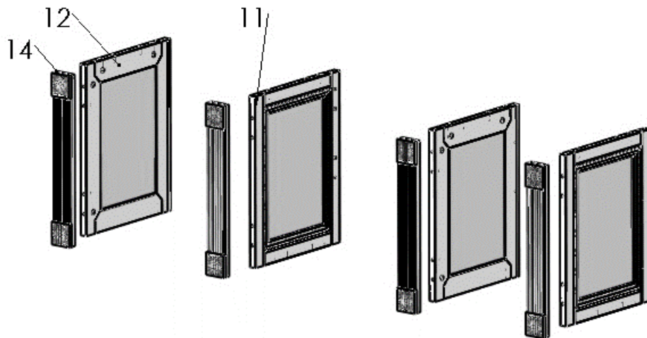
Рисунок 2 – Сборка пилястр со стенками тумб
