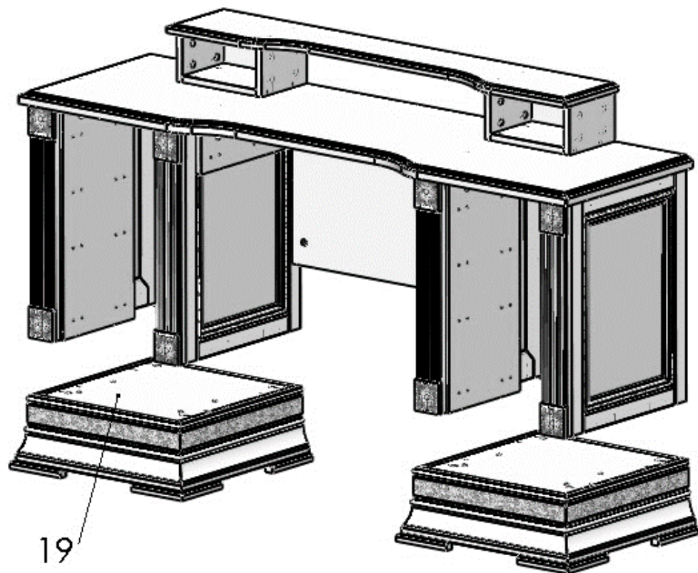
Рисунок 5 – Крепление подиумов к стенкам тумб
