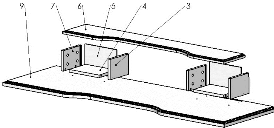
Рисунок 1 – Сборка элементов полки
