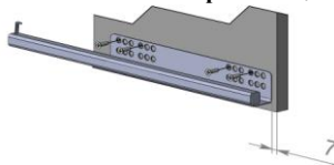
Установка направляющих
