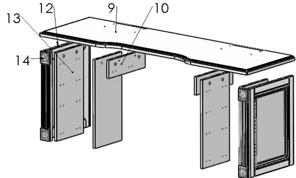
Рисунок 4 – Сборка вертикальных стенок тумб со столешницей
