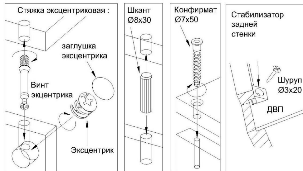
Схема основных крепежных узлов
