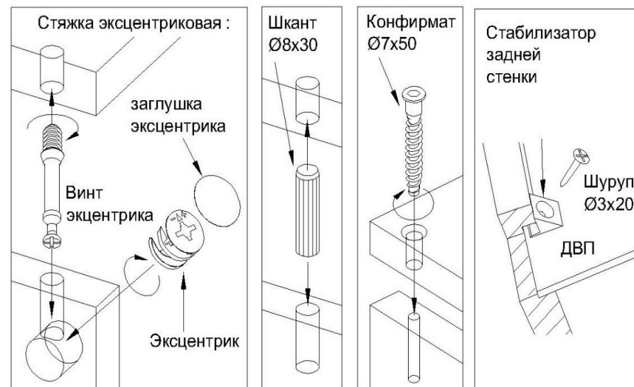
Схема основных крепежных узлов
