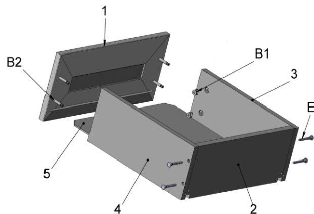
Схема сборки ящика выдвижного
